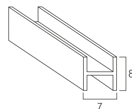
Blindatura per av. 7 x 8 mm
