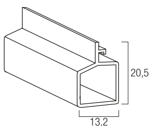
Terminale Pvc Super 13,2 x 20,5 mm
