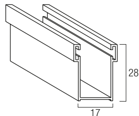
Guida in alluminio A28 17 x 28 mm
