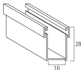
Guida in alluminio A16 16 x 28 mm
