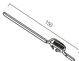
Catenacciolo per terminale 150 mm
