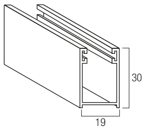
Guida in alluminio A19 19 x 30 mm
