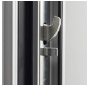
SERRATURA MECCANICA CON INCONTRI SCIOLTI + GANCI E PUNZONI A 3 PUNTI
